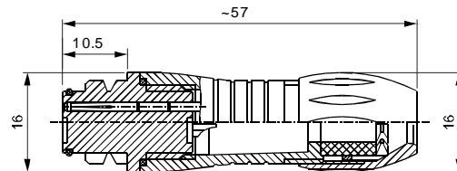
电缆插头, 电缆直径 4-6mm 针数 3,5,8
