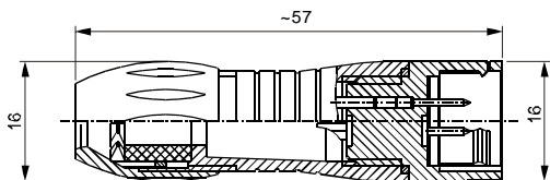
电缆插头, 电缆直径 4-6mm 针数 3,5,8
